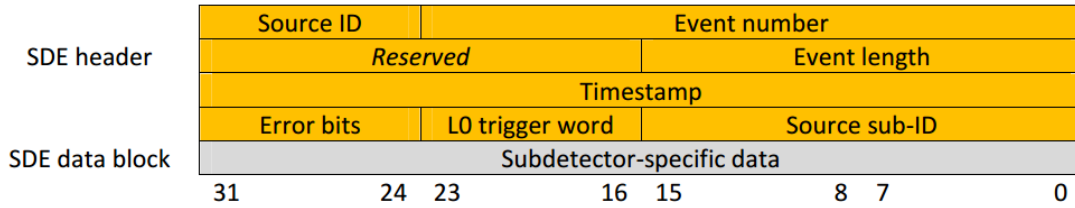
Figure 4.4: SDE format.
