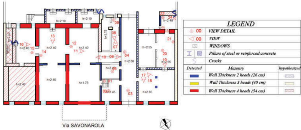
FIG. 5. Basement plan.
