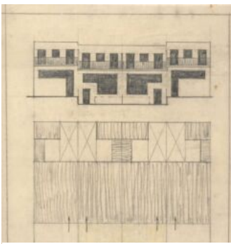
Adolf Loos, Casa dopp...
